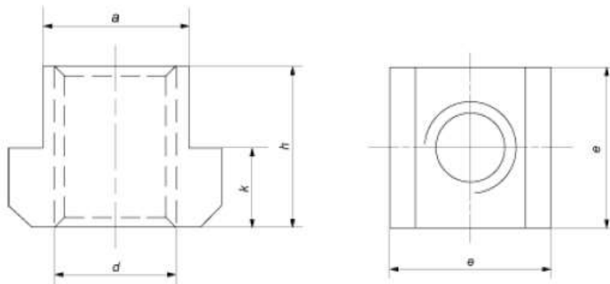
Гайка для Т-образных пазов DIN 508 (ISO 299)
